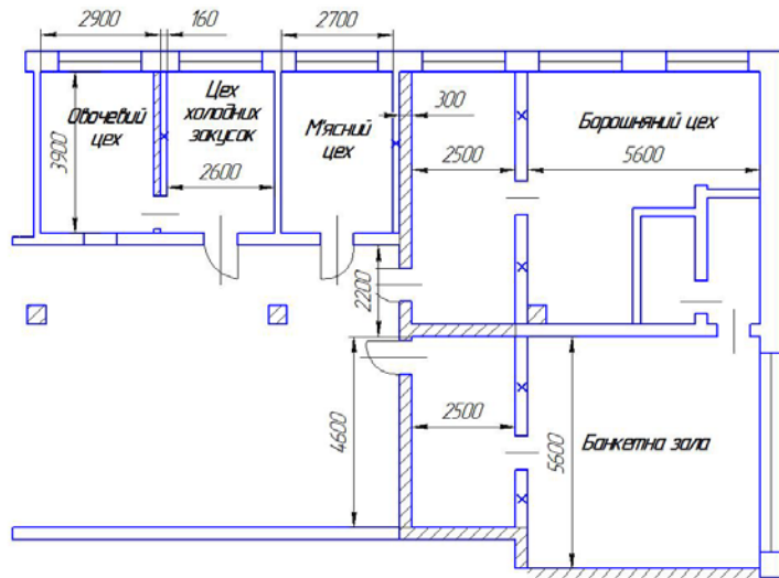
План реконструкції кухні їдальні НАТІ
